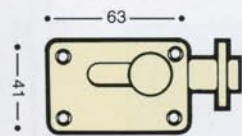
0448 DOOR BOLT • knob slide action
