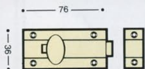
0448 DOOR BOLT • knob slide action
